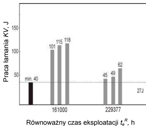
Rysunek 43. Wpływ długotrwałej eksploatacji w warunkach pełzania na udarność w temperaturze pokojowej materiału komory przegrzewacza pary części ciśnieniowej kotłów energetycznych wykonanych z niskostopowej stali 16Mo3; T_e^R = 500^\circ\text{C}
