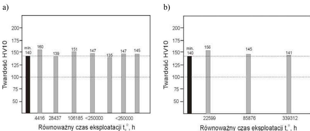
Rysunek 53. Wpływ długotrwałej eksploatacji w warunkach pełzania na twardość materiału elementów krytycznych kotła z niskostopowej stali 10CrMo9-10: a) węzłowniczka przegrzewacza pary, b) komór przegrzewacza pary i rurociągów pary wtórnej: T_e^R = 540^\circ\text{C}
