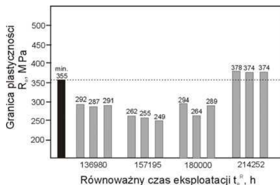
Rysunek 31. Wpływ długotrwałej eksploatacji w warunkach pełzania materiału wycinków głównych rurociągów pary świeższej kotłów energetycznych z niskostopowej stali 14MoV6-3 na granicę plastyczności w temperaturze pokojowej; T_e^R = 540^\circ\text{C}
