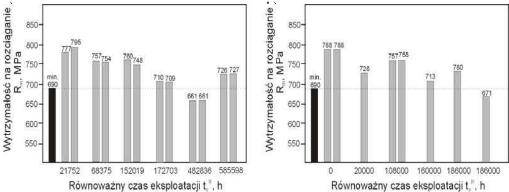
Rysunek 27. Wpływ długotrwałej eksploatacji w warunkach pełzania materiału elementów części ciśnieniowej kotłów energetycznych z wysokochromowej stali X20CrMoV11-1 na wytrzymałość na rozciąganie w temperaturze pokojowej; a) węzłowiec przegrzewacza pary; T_e^R = 570^\circ\text{C} , b) komór wylotowych przegrzewacza pary; T_e^R = 540^\circ\text{C}
