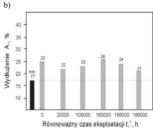
Rysunek 37. Wpływ długotrwałej eksploatacji w warunkach pełzania materiału elementów kotłów energetycznych z wysokochromowej stali X20CrMoV11-1 na wydłużenie w próbie rozciągania w temperaturze pokojowej: a) węzownic przegrzewacza pary; T_e^R = 570^\circ\text{C} , b) komór przegrzewacza pary; T_e^R = 540^\circ\text{C}
