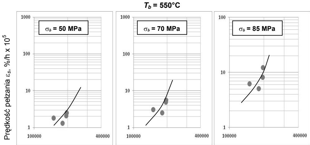
Rysunek 72b. Prędkość pelzania w stanie stacjonarnym \dot{\epsilon}_s w funkcji równoważnego czasu eksploatacji t_e^R przy stałym poziomie naprężenia \sigma materiałów wycinków głównych rurociągów pary świeżej kotłów energetycznych z niskostopowej stali 14MoV6-3 po eksploatacji poza obliczeniowy czas pracy w temperaturze 550^\circ\text{C} dalszej eksploatacji (równoważna temperatura eksploatacji T_e^R = 540^\circ\text{C} )
