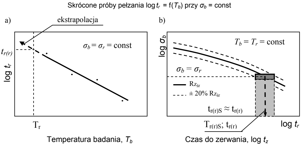
Rysunek 57. Wiarygodność oszacowania czasu do zerwania t_r dla parametrów roboczych w oparciu o wyniki skróconych prób pełzania przy stałym naprężeniu badania odpowiadającym roboczemu \sigma_b = \sigma_r = \text{const} ;
