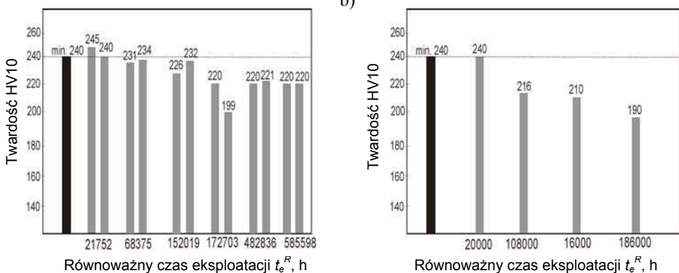
Rysunek 55. Wpływ długotrwałej eksploatacji w warunkach pełzania na twardość materiału elementów przegrzewaczy pary z wysokochromowej stali X20CrMoV11-1: a) wężownicz; T_e^R = 570^\circ\text{C} , b) komór wylotowych; T_e^R = 540^\circ\text{C}
