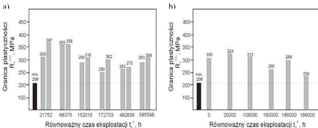
Rysunek 42. Wpływ długotrwałej eksploatacji w warunkach pełzania materiału elementów kotłów energetycznych z wysokochromowej stali X20CrMoV11-1 na granicę plastyczności w podwyższonej temperaturze: a) węzownic przegrzewacza pary; T_e^R = 570^\circ\text{C} , b) komór przegrzewacza pary; T_e^R = 540^\circ\text{C}
