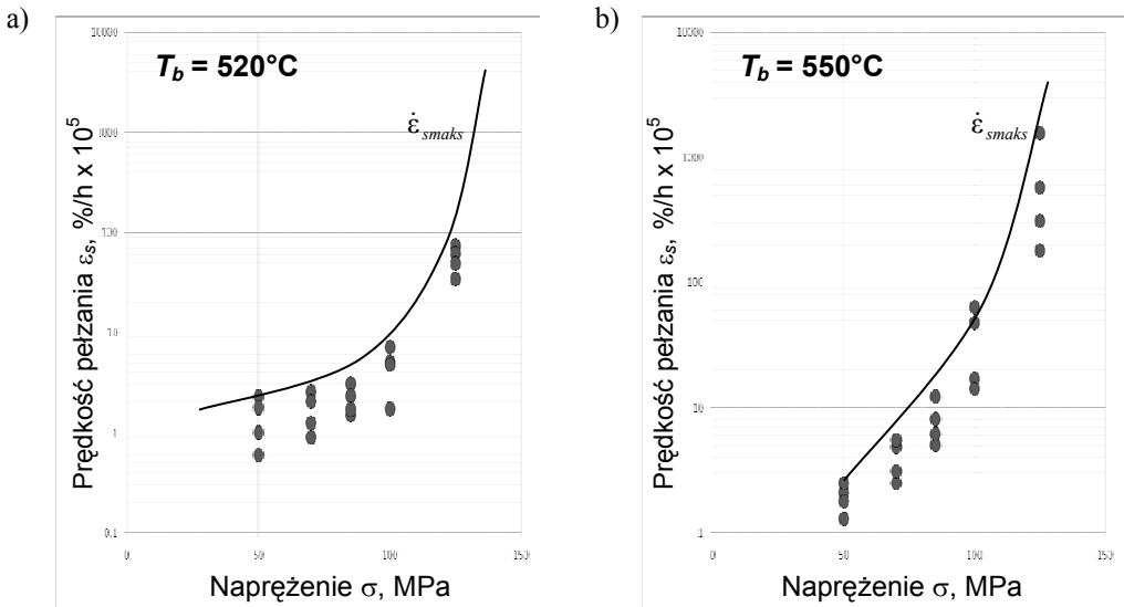
Rysunek 73. Maksymalna prędkość pelzania w stanie stacjonarnym \dot{\epsilon}_s w zależności od naprężenia \sigma materiałów wycinków głównych rurociągów pary świeżej kotłów energetycznych z niskostopowej stali 14MoV6-3 po eksploatacji poza obliczeniowy czas pracy dla temperatury dalszej eksploatacji: a) 520^\circ\text{C} , b) 550^\circ\text{C}
