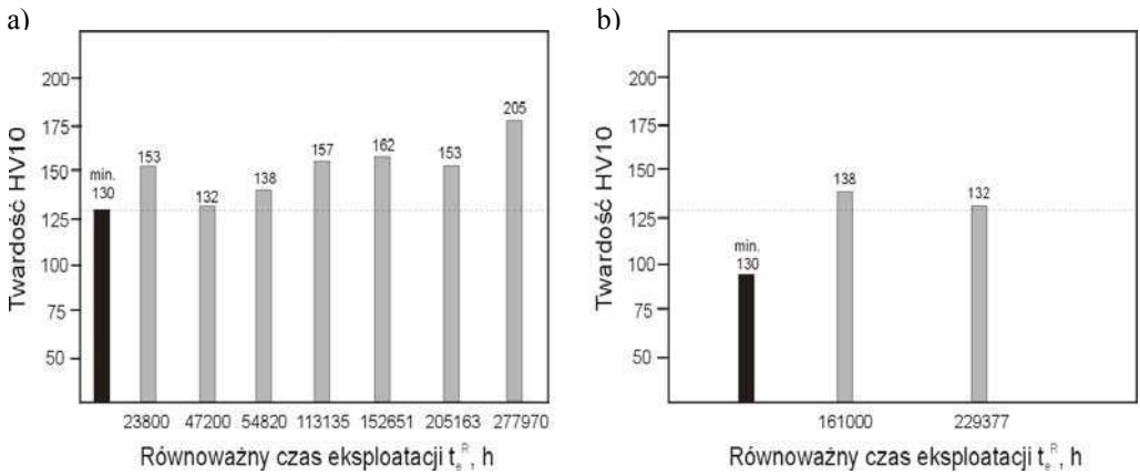
Rysunek 51. Wpływ długotrwałej eksploatacji w warunkach pełzania na twardość materiału elementów krytycznych kotła z niskostopowej stali 16Mo3: a) wężownica przegrzewacza pary, b) komór przegrzewacza pary; T_e^R = 500^\circ\text{C}
