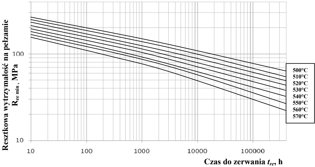
Rysunek 65. Charakterystyki minimalnej resztkowej czasowej wytrzymałości na pełzanie w postaci zależności \log \sigma_b = f(\log t_r) dla różnych poziomów przewidywanej temperatury dalszej eksploatacji niskostopowej stali 13CrMo4-5 po eksploatacji poza obliczeniowy czas pracy o niezapoczątkowanym procesie wewnętrznych uszkodzeń
