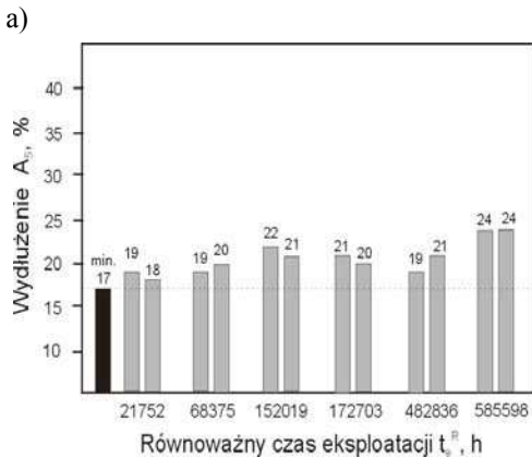
Rysunek 37. Wpływ długotrwałej eksploatacji w warunkach pełzania materiału elementów kotłów energetycznych z wysokochromowej stali X20CrMoV11-1 na wydłużenie w próbie rozciągania w temperaturze pokojowej: a) węzownic przegrzewacza pary; T_e^R = 570^\circ\text{C} , b) komór przegrzewacza pary; T_e^R = 540^\circ\text{C}
