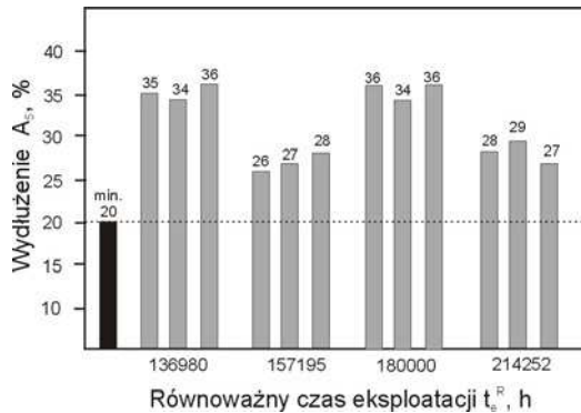
Rysunek 36. Wpływ długotrwałej eksploatacji w warunkach pełzania materiału wycinków głównych rurociągów pary świeżej kotłów energetycznych z niskostopowej stali 14MoV6-3 na wydłużenie w próbie rozciągania w temperaturze pokojowej; T_e^R = 540^\circ\text{C}
