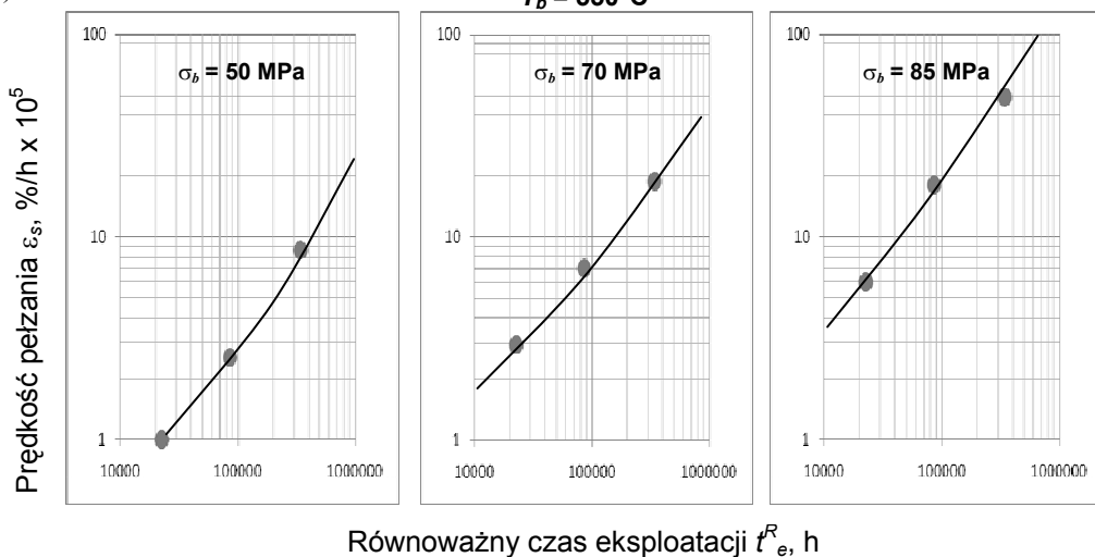
Rysunek 70. Prędkość pelzania w stanie stacjonarnym \dot{\epsilon}_s w funkcji równoważnego czasu eksploatacji t_e^R przy stałym poziomie naprężenia \sigma materiałów elementów części ciśnieniowej kotła po eksploatacji poza obliczeniowy czas pracy wykonanych z niskostopowej stali 10CrMo9-10 w temperaturze dalszej eksploatacji: a) 520^\circ\text{C} , b) 550^\circ\text{C} (równoważna temperatura eksploatacji T_e^R = 540^\circ\text{C} )
