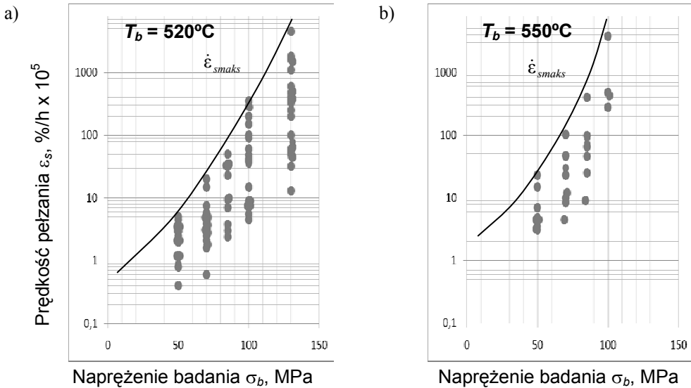
Rysunek 69. Maksymalna prędkość pełzania w stanie stacjonarnym \dot{\epsilon}_{s_{maks}} w zależności od naprężenia badania \sigma_b materiałów elementów komór przegrzewaczy pary kotła po eksploatacji poza obliczeniowy czas pracy wykonanych z niskostopowej stali 13CrMo4-5 dla temperatury dalszej eksploatacji: a) 520^\circ C , b) 550^\circ C (równoważna temperatura eksploatacji T_e^R = 520^\circ C )
